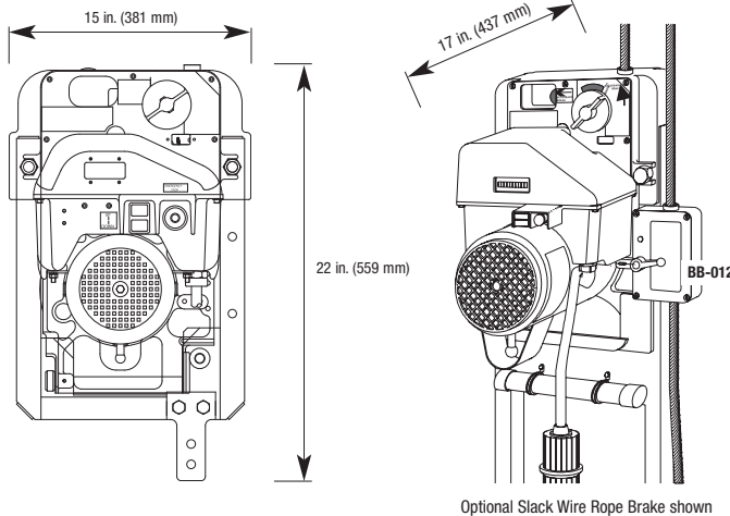
Optional Slack Wire Rope Brake shown
